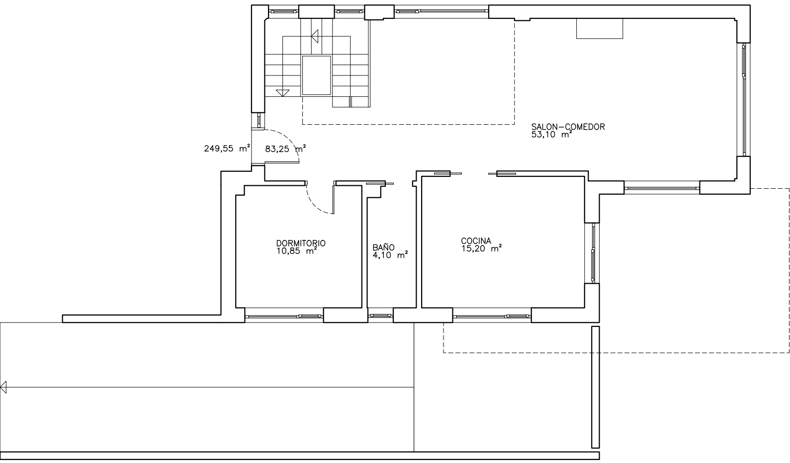
PLANTA BAJA
