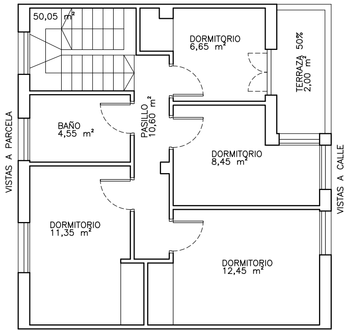
PLANTA ALTA
