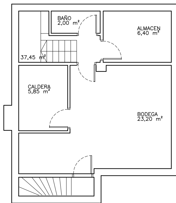
PLANTA SOTANO
