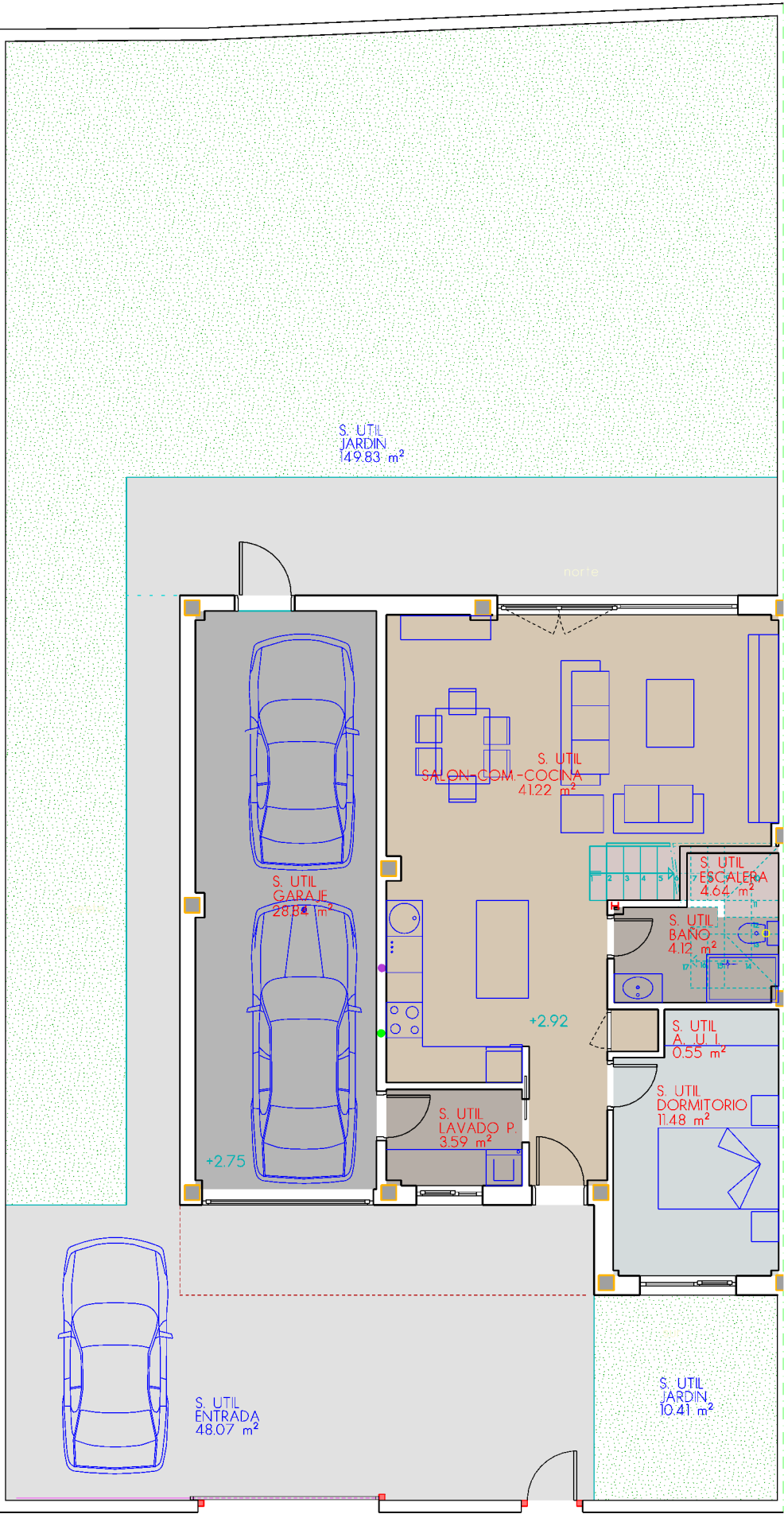
PLANTA BAJA
