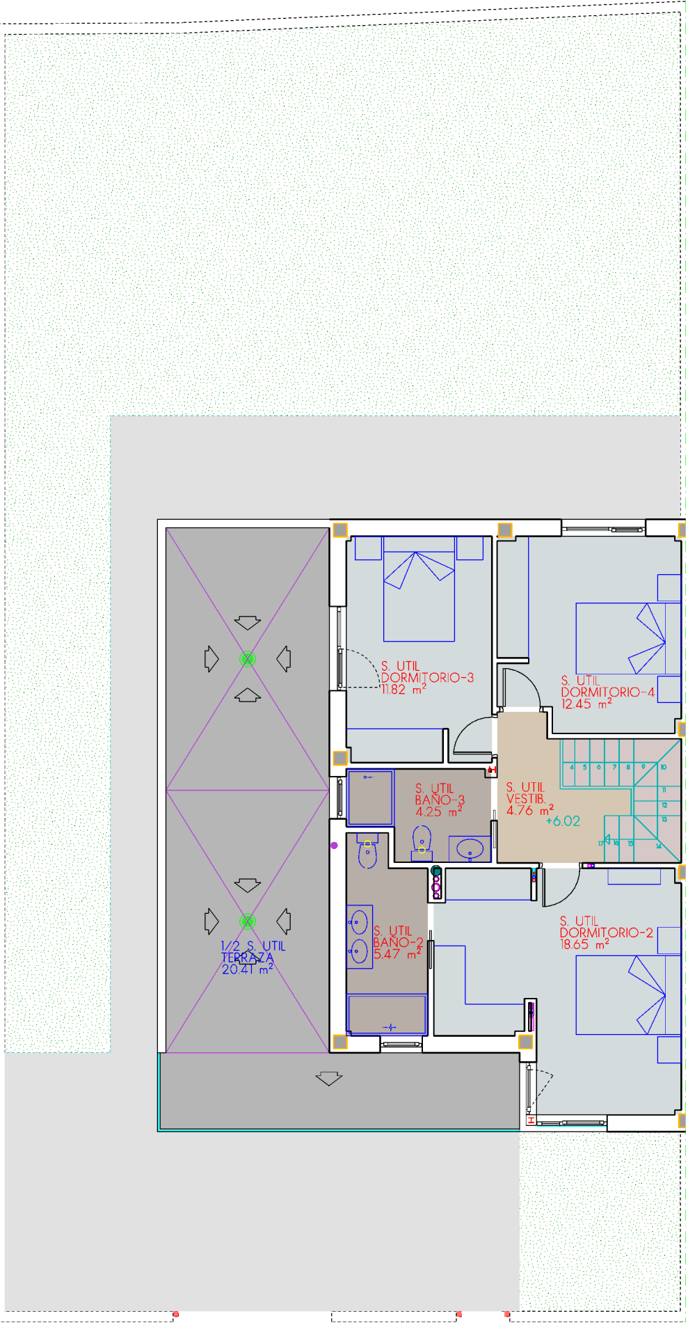
PLANTA PRIMERA
